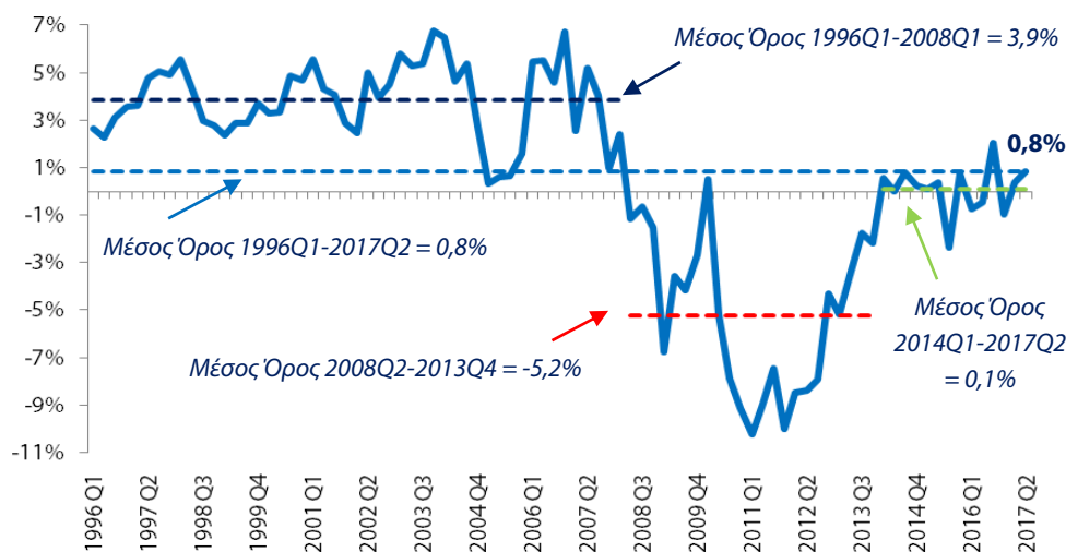
Σχήμα 1: Ετήσια % Μεταβολή του Πραγματικού ΑΕΠ, 1996Q1-2017Q2 (%)
