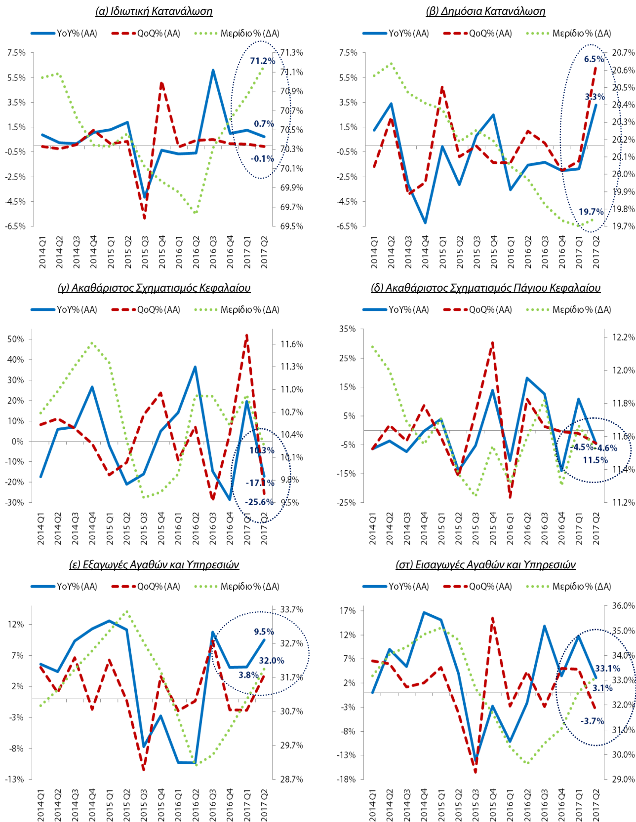
Σχήμα 2: Συνιστώσες του Πραγματικού ΑΕΠ – Προσέγγιση Δαπάνης, Ετήσια % Μεταβολή (YoY%), Τριμηνιαία % Μεταβολή (QoQ%) και Μεριδία Επί του Συνόλου του ΑΕΠ (%)
